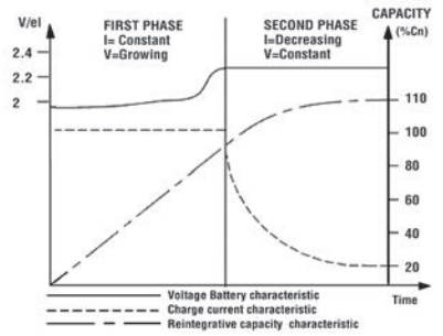
PROFILO DI RICARICA / CHARGE PROFILE IU (Norme / Standards DIN 41773)
