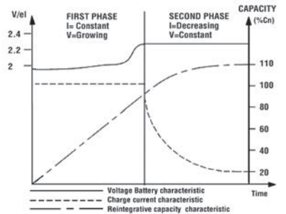
PROFILO DI RICARICA / CHARGE PROFILE IU (Norme / Standards DIN 41773)
